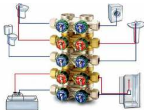
Рис. 76 Колектор для холодного та гарячого водопостачання в одній шафі
