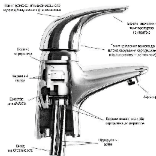
Рис. 36 Загальна будова змішувача води (одноважільний)
