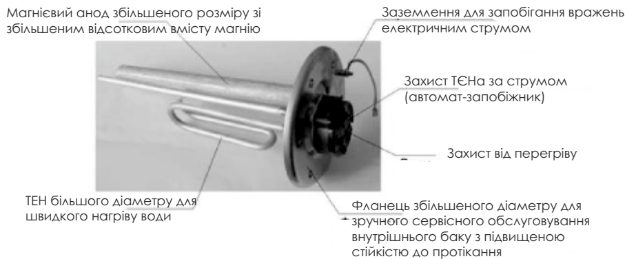
Рис. 109 ТЕН в зборі
