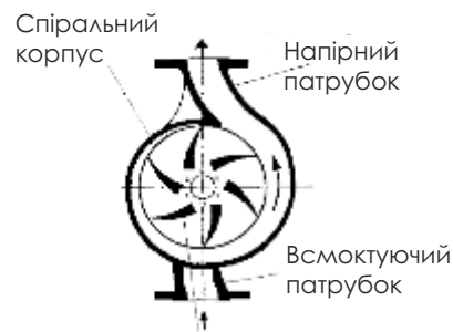
Рис. 56 Крильчатка з викривленими назад лопастями
