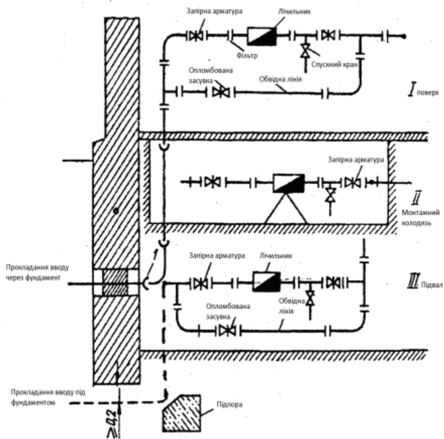
Рис. 22 Приклад вводу через фундамент і під фундаментом
