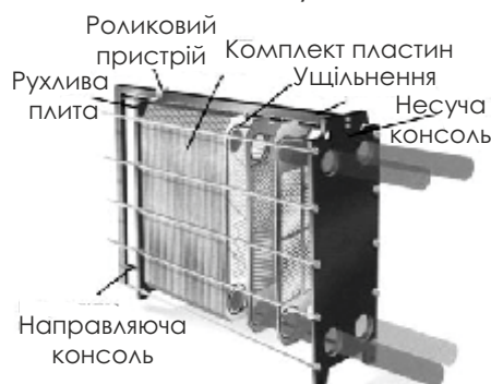
Рис. 98 Швидкісний пластинчатий водонагрівач
