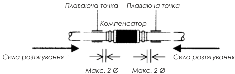
Рис. 81 Схема компенсатора
