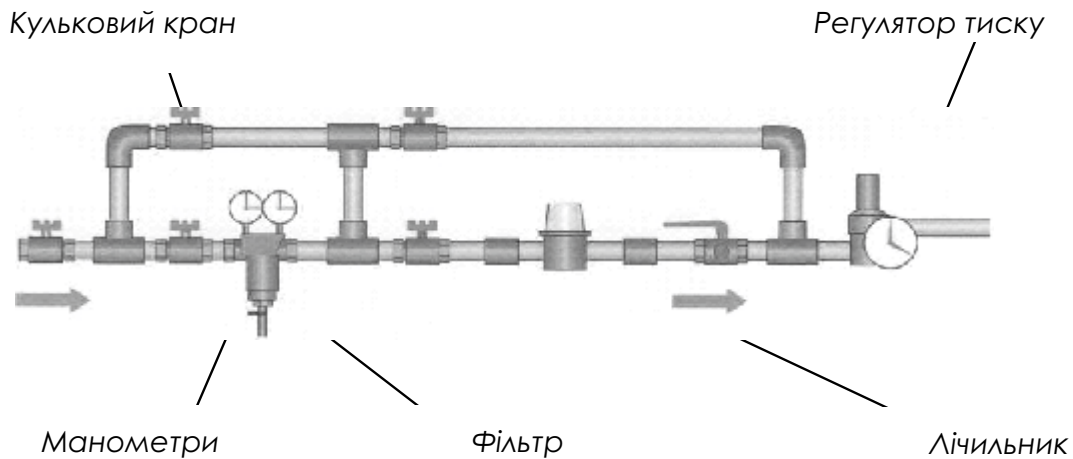
Рис. 21 Схема вузла з регулятором тиску
