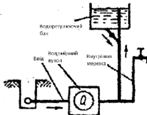
Рис. 15 Схема з регулюючими баками
