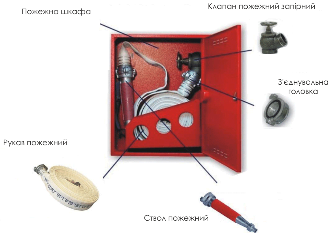
Рис. 67 Пожежна шафа
