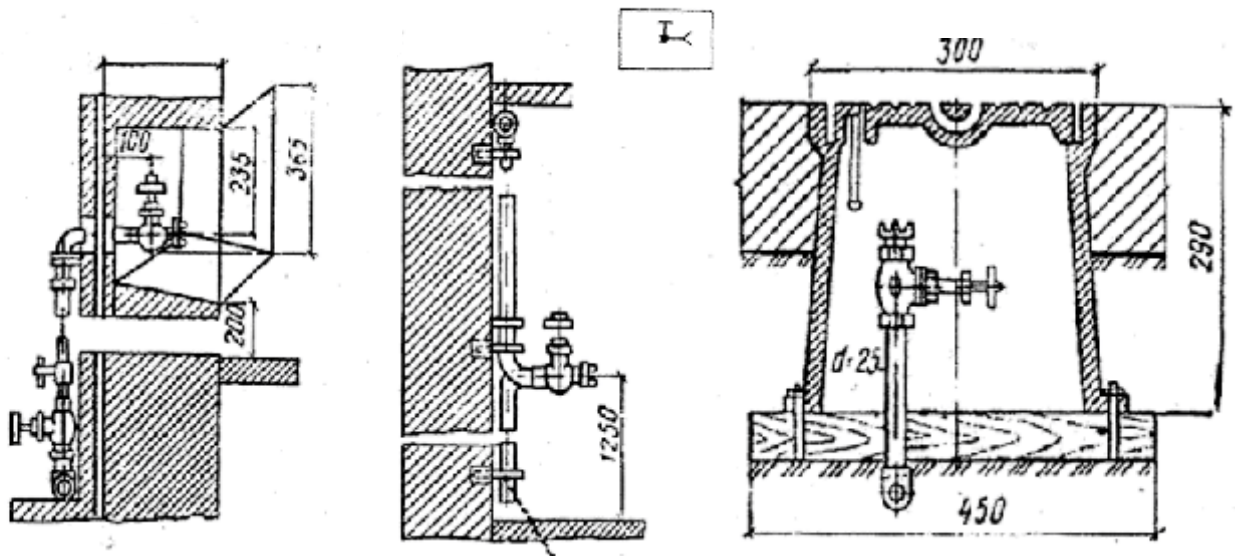
Рис. 69 Поливальний кран
