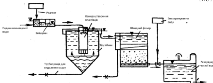
Рис. 6 Схема очисної станції при очищенні з реагентами
