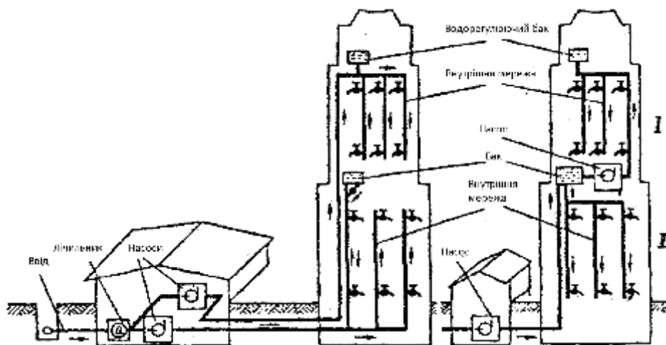
Рис. 18 Схеми зонного водопроводу
