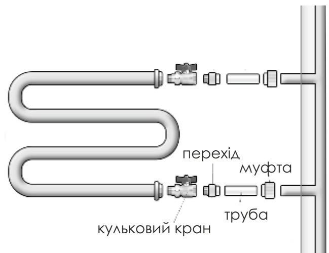
Рис. 111 Монтаж рушникосушія
